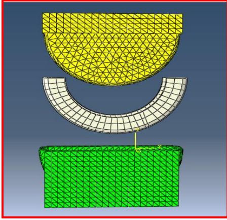
"Fig. 5". Meshed assembly
